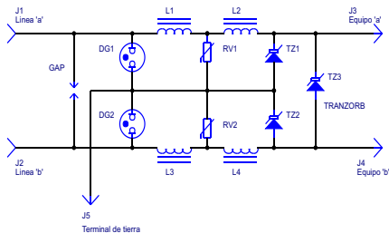
Figura 1. Diagrama interno G-Ray
